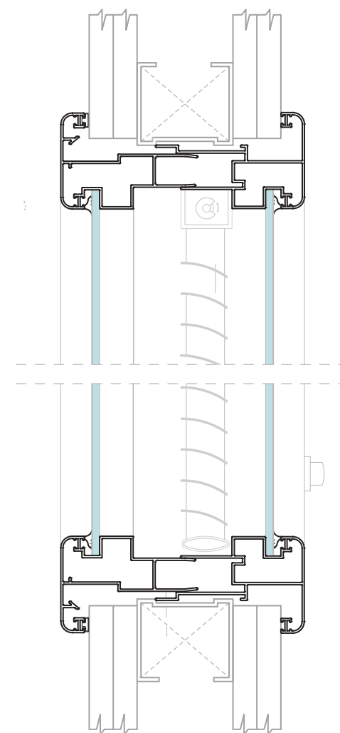
Τοιχοποιία 100mm
