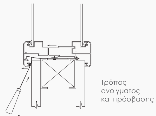
Λεπτομέρεια 3
