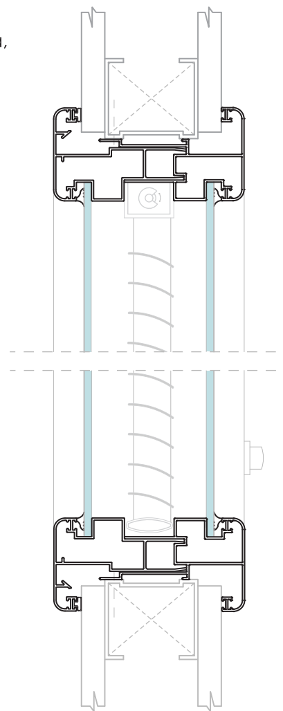
Τοιχοποιία 75mm
