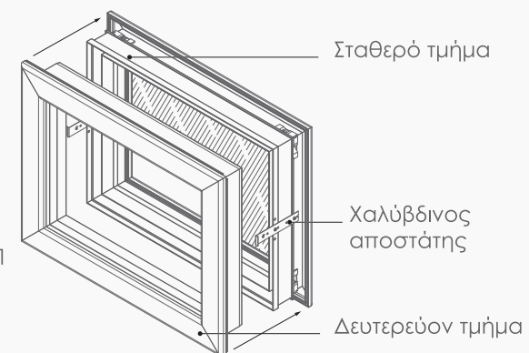
Λεπτομέρεια 1
