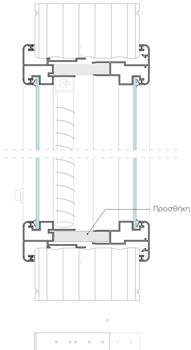
Λεπτομέρεια 1
