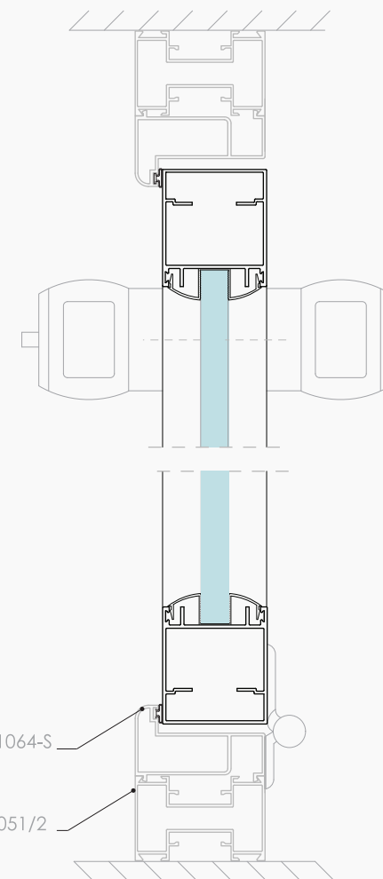
Οριζόντια τομή
